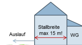
Abb. 2: Beispielskizze Stallbreite
